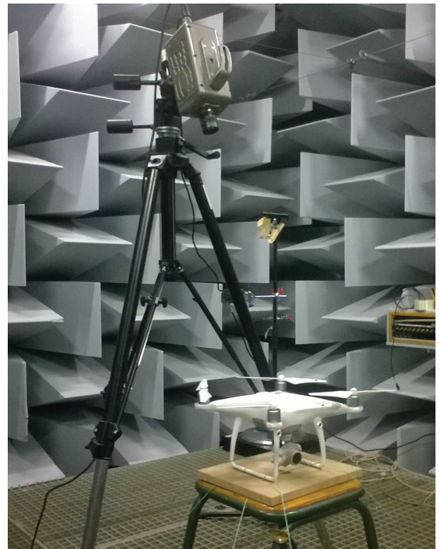
FIGURE 4 – Photo du drone fixé en 8 points d'attaches à l'aide de fils en nylon. La caméra rapide pointée verticalement au-dessus du drone permet de mesurer la vitesse de rotation des hélices.
