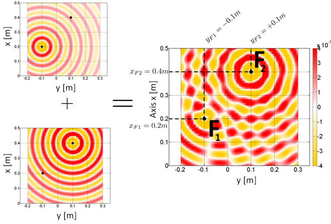
FIGURE 4 – Champ de déplacement \bar{w}_{sum}(x, y) d'une plaque infinie excitée par 2 forces harmoniques F_1 et F_2 (partie réelle). Le côté droit est la somme des contributions \bar{w}_{F1}(x, y) (en haut à gauche) et \bar{w}_{F2}(x, y) (en bas à gauche) produite respectivement par les forces F_1 et F_2
