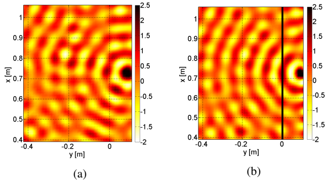
FIGURE 8 – (a) Déplacement référence et (b) déplacement reconstruit par FSH. Le trait noir plein vertical représente la position des hologrammes.
