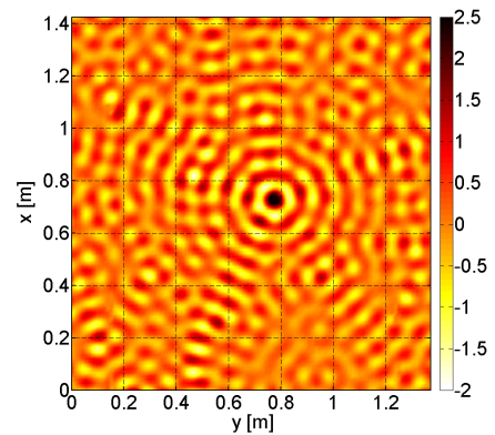
FIGURE 7 – Mesure directe du champ de déplacement d'une plaque d'aluminium excitée par un pot-vibrant avec un signal pseudo aléatoire à la fréquence f = 1418 Hz.
