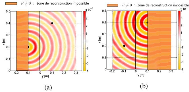
FIGURE 5 – Déplacement reconstruits (a) w_{F1}^{rec}(x, y) et (b) w_{F2}^{rec}(x, y) calculés avec l'Eq.(8). Le trait vertical indique la position des hologrammes ( y_h = 0 et 0.01 m).
