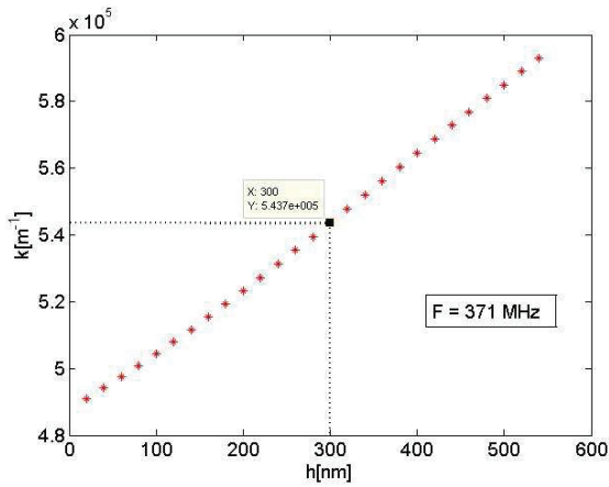
FIGURE 14 – Influence de l'épaisseur du bicouche Ni/Cu sur le nombre d'onde à une fréquence F = 371 MHz.
