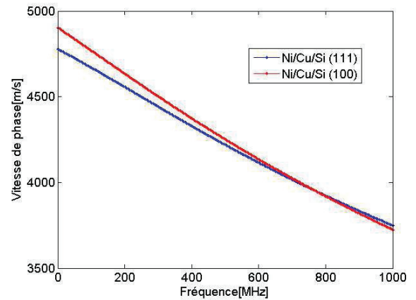
FIGURE 2 – vitesse de phase de premier mode Rayleigh dans des multicouche Ni/Cu/Si.
